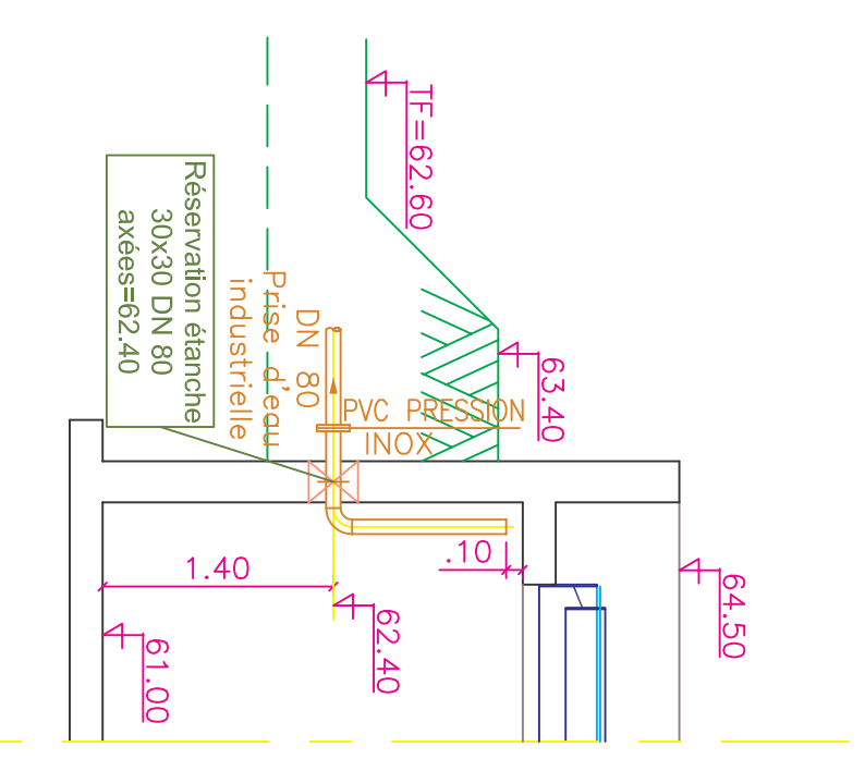
COUPE JJ Echelle: 1/50
