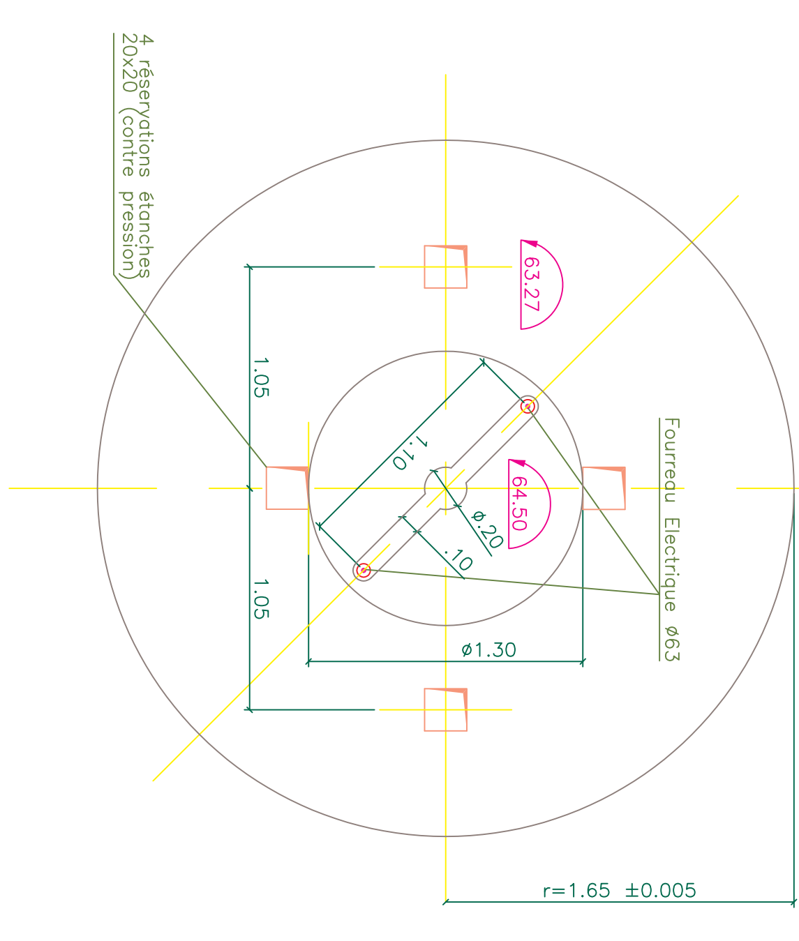
COUPE EE Echelle: 1/25
