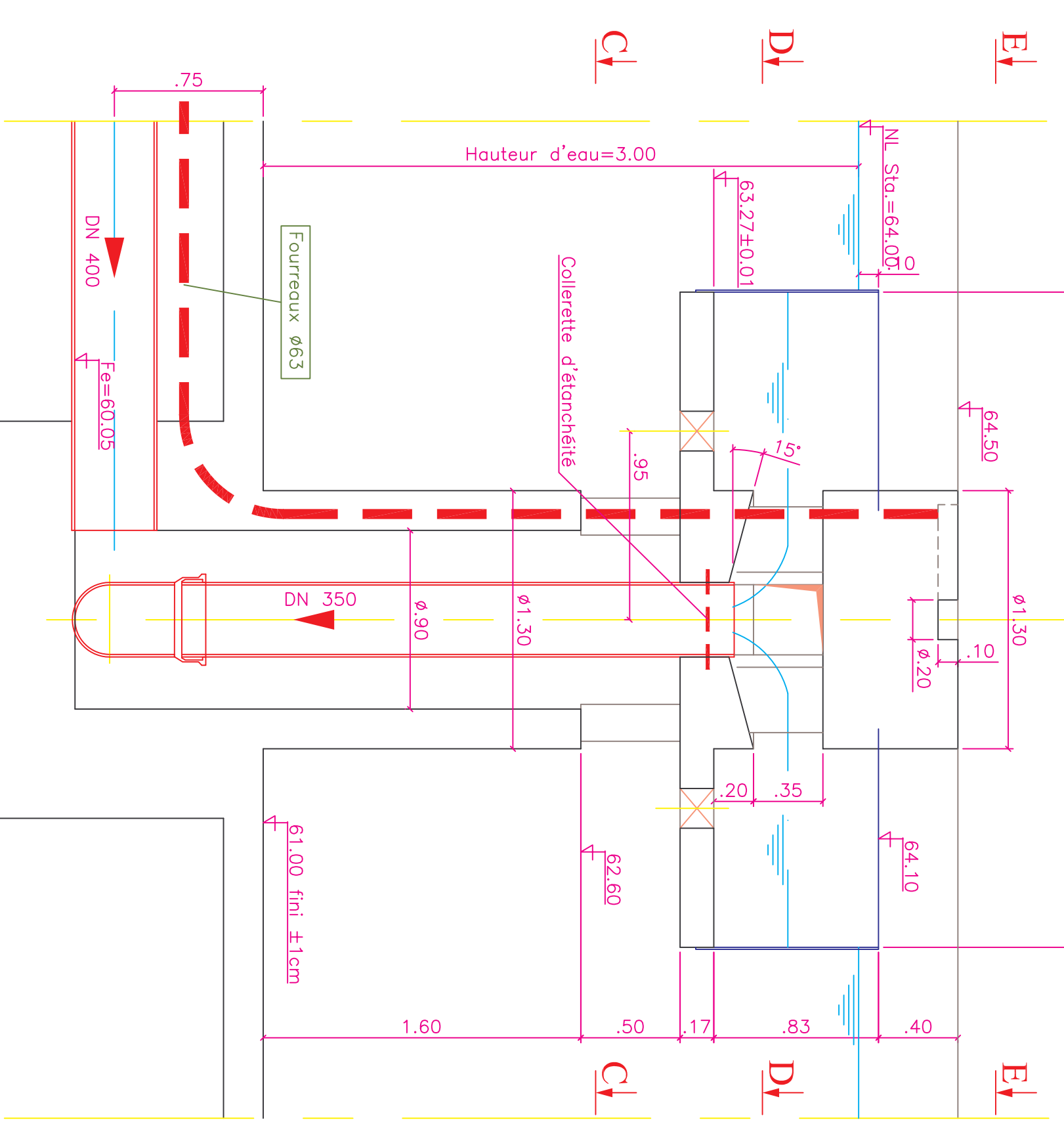
COUPE BB Echelle: 1/25
